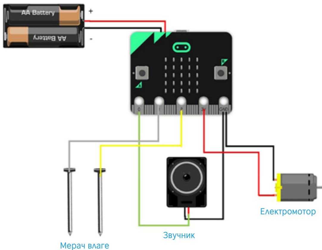
Шема повезивања са микробитом
